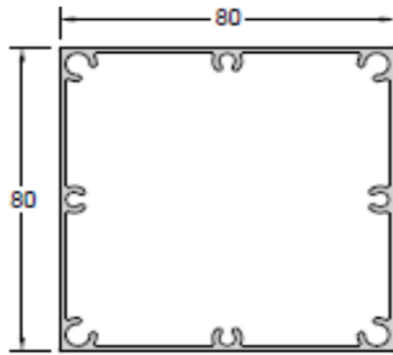
Pfosten 80x80 gewicht: 1606 gr/m
