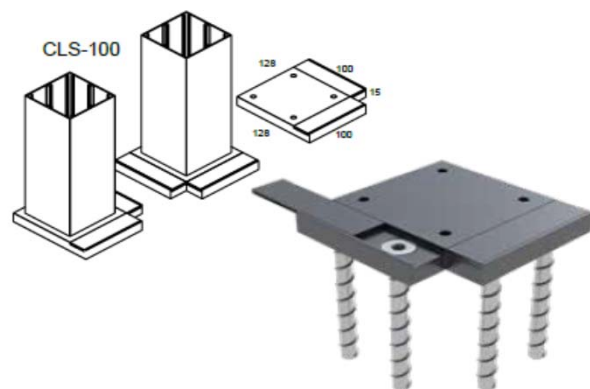
Aufgesetzte Eckverankerung für den Pfosten CLS 100 128x100x128x100x15 incl. 4 x Schrauben
