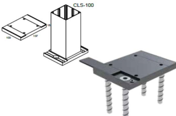
Aufgesetzte Verankerung für den Pfosten CLS 100 100x137x15 incl. 4 x Schrauben
