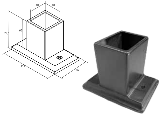
Code: G4113 Fußpunkt für Pfosten 40x40
