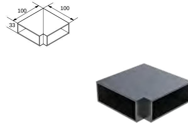
Code: 4273 Eckverbinder Handlauf CLS-201/FSN-221
