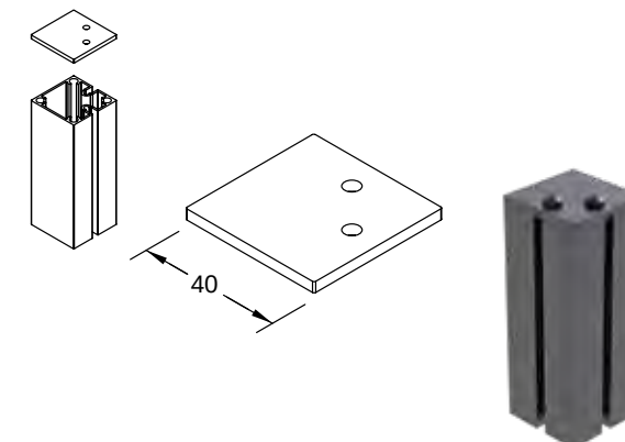
Code: 4490 DECKEL FÜR PFOSTEN CLS-104 (40x40) FLAT
