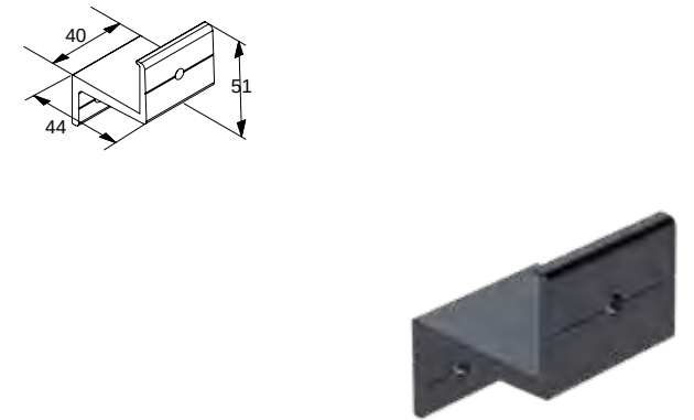
Code: G4274 GURTHALTER FÜR GELÄNDERMATTEN
