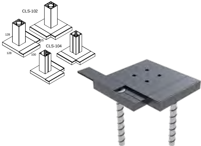
Code: 4724 ECKVERANDERUNG FÜR PFOSTEN 40x40 CLS-102
