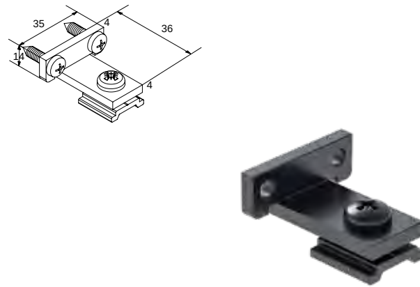
Code: G4270 VERBINDER FÜR CLS-201/301/302/305
