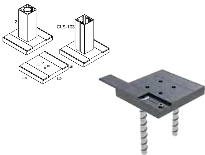
Code: 4723 VERANKERUNG FÜR PFOSTEN 40x40 CLS-102
