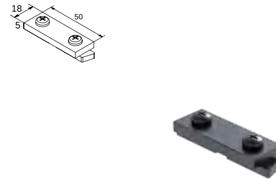
Code: 4275 VERBINDER FÜR GURT CLS-302
